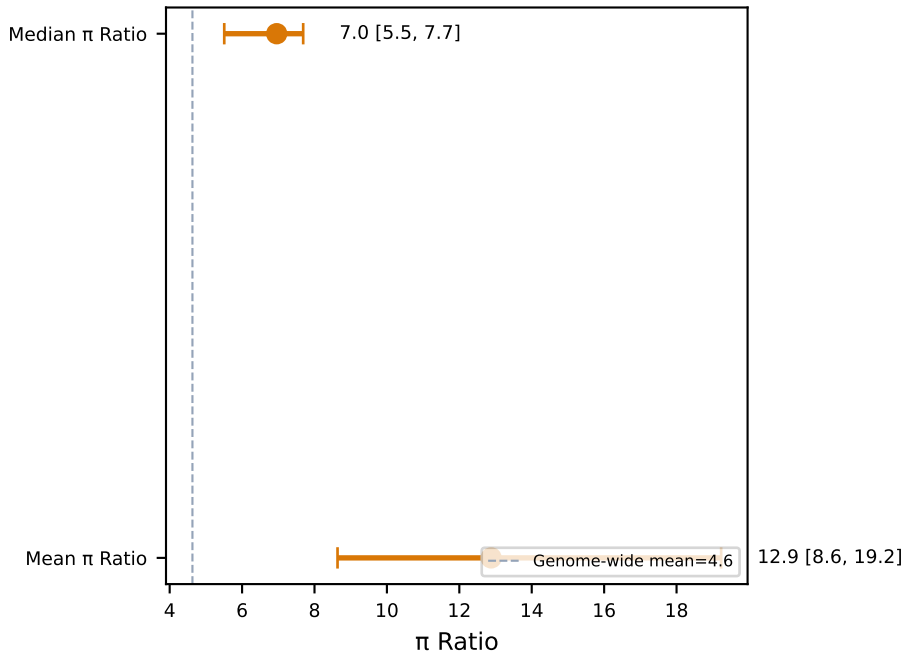
A: Bootstrap 95% CI (n=10,000 resamples)
